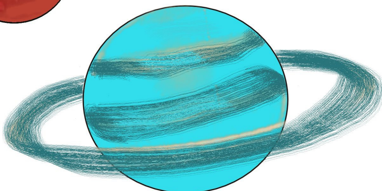
Uranus
