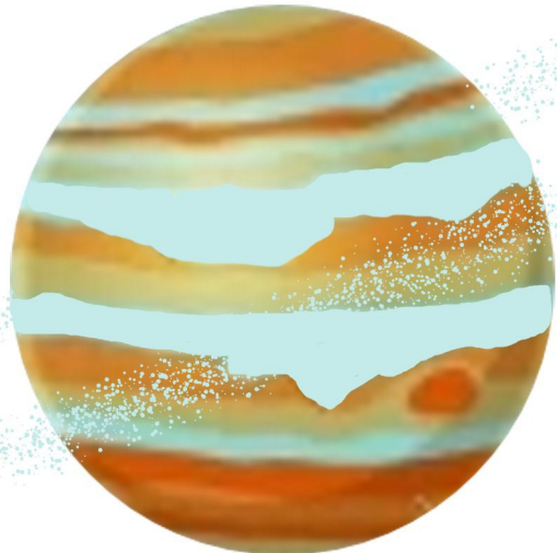
Jupiter
